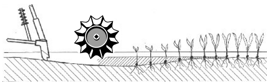
Послепосевная прокатка, неравномерная глубина посева, замедленные всходы.
